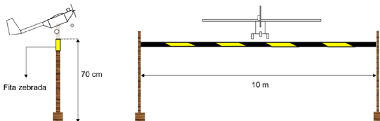
Figura 8.4: Decolagem válida Classe Advanced : obstáculo.
