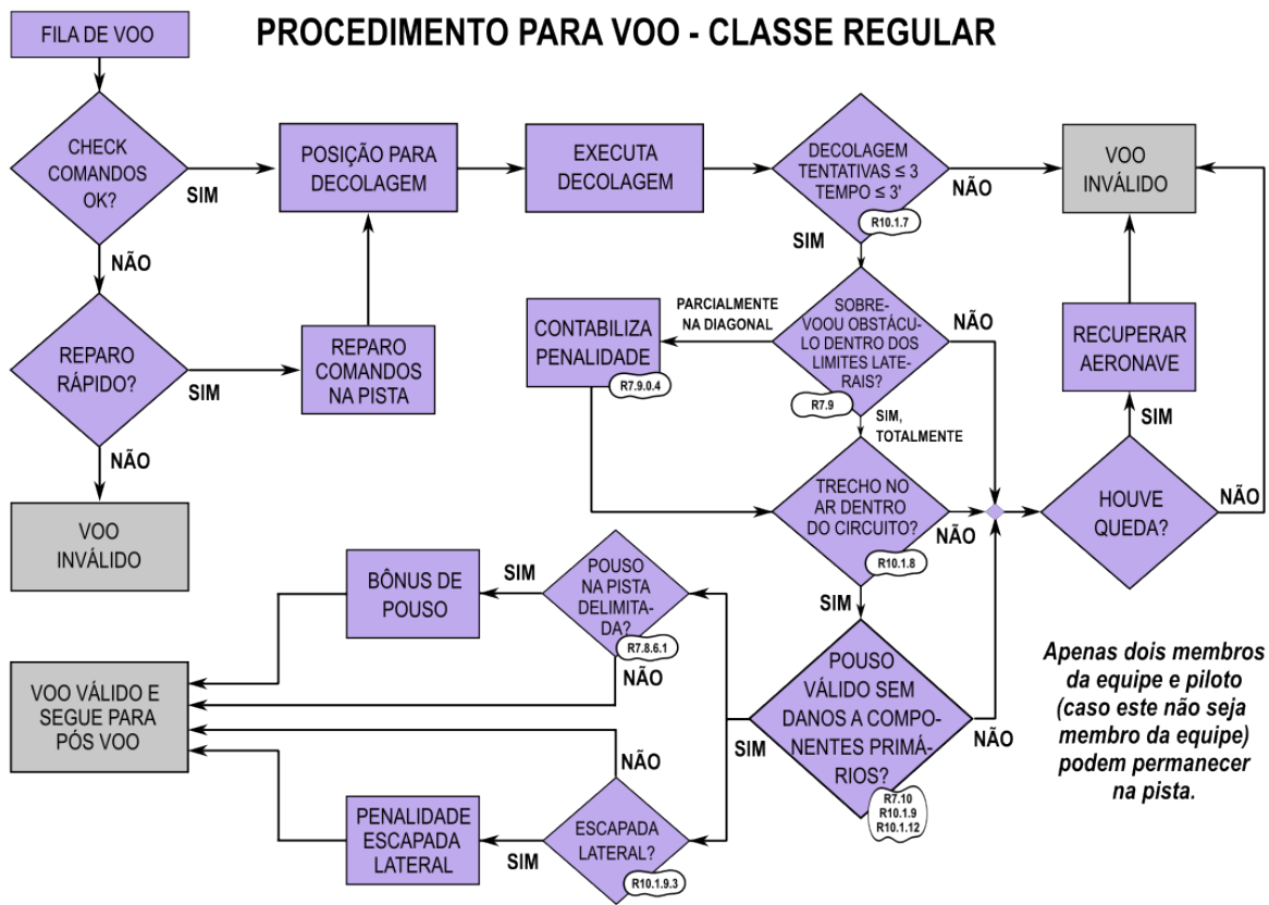
Figura 15.5: Voo - Classe Regular
