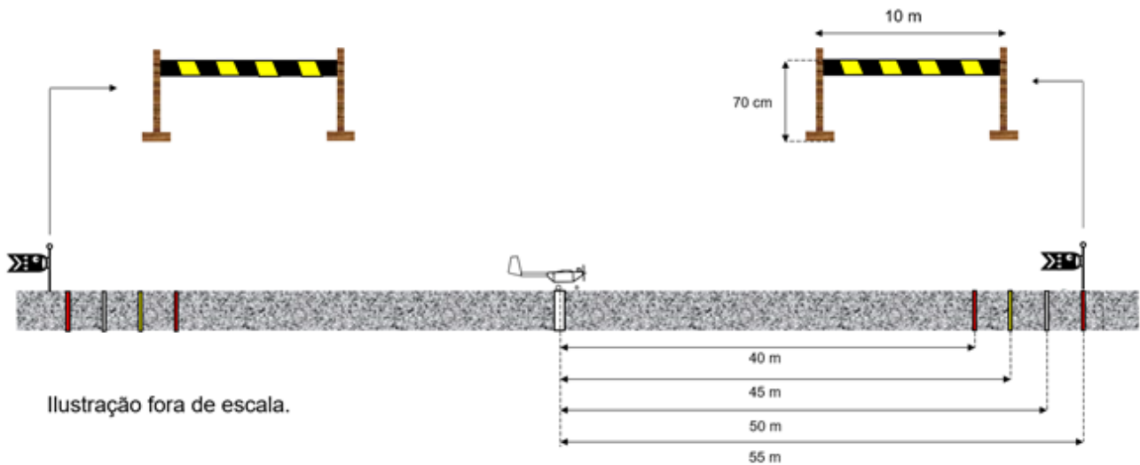
Figura 8.5: Decolagem válida Classe Advanced : pista com obstáculo.
