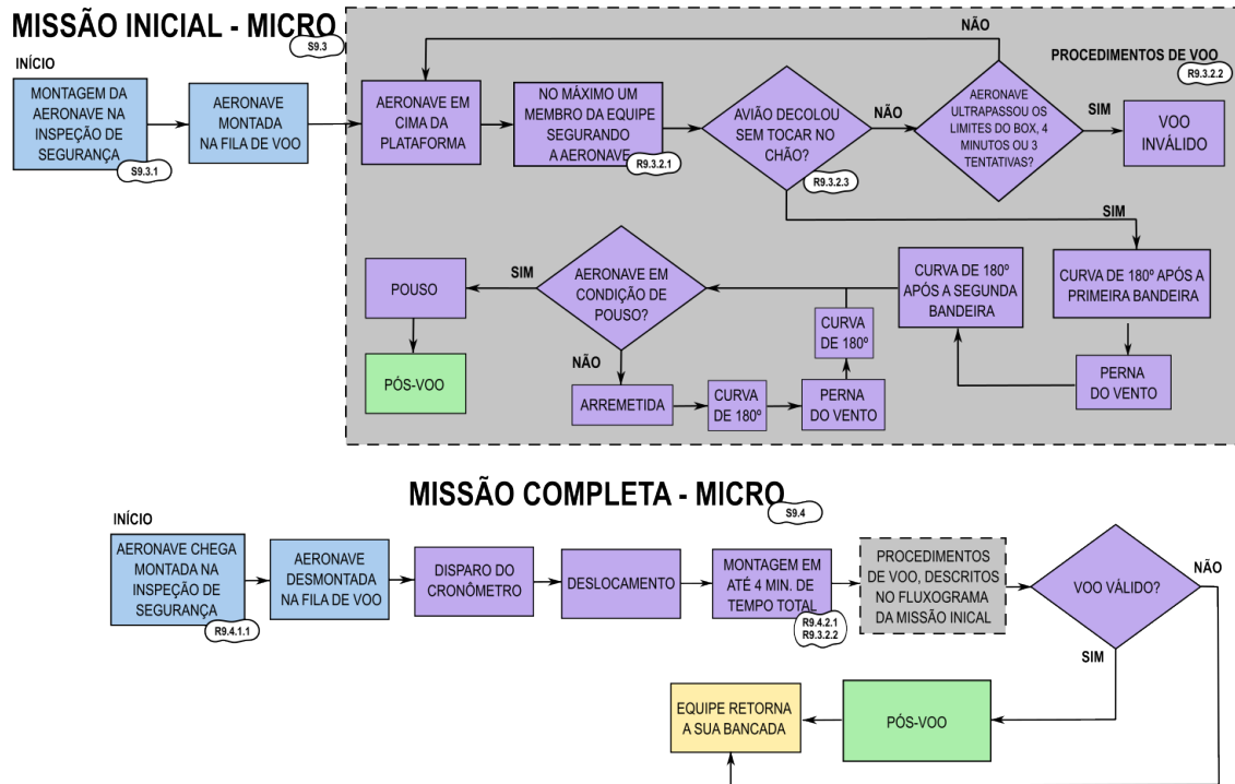
Figura 15.7: Voo - Classe Micro
