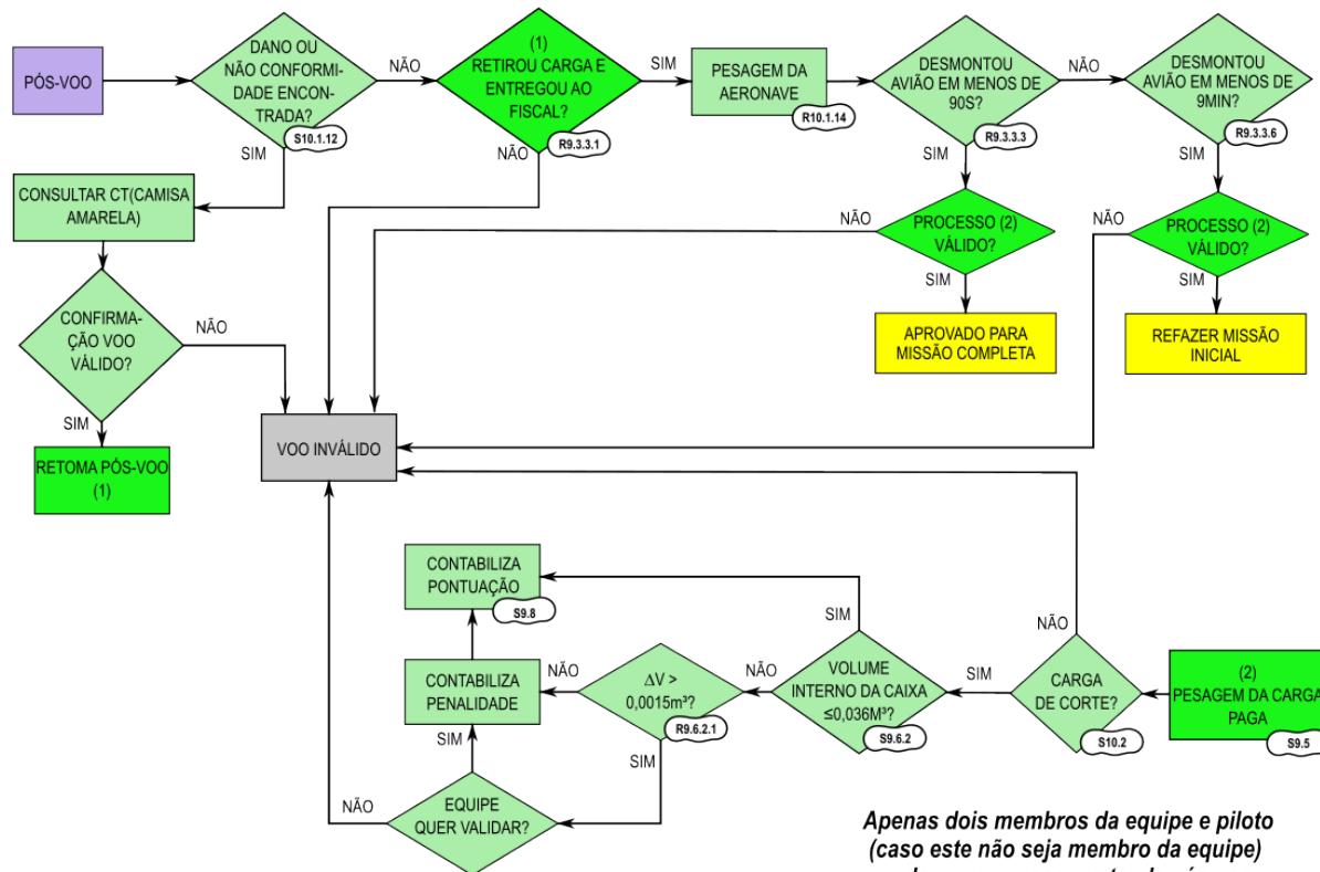
Figura 15.8: Pós-Voo Missão Inicial - Classe Micro
