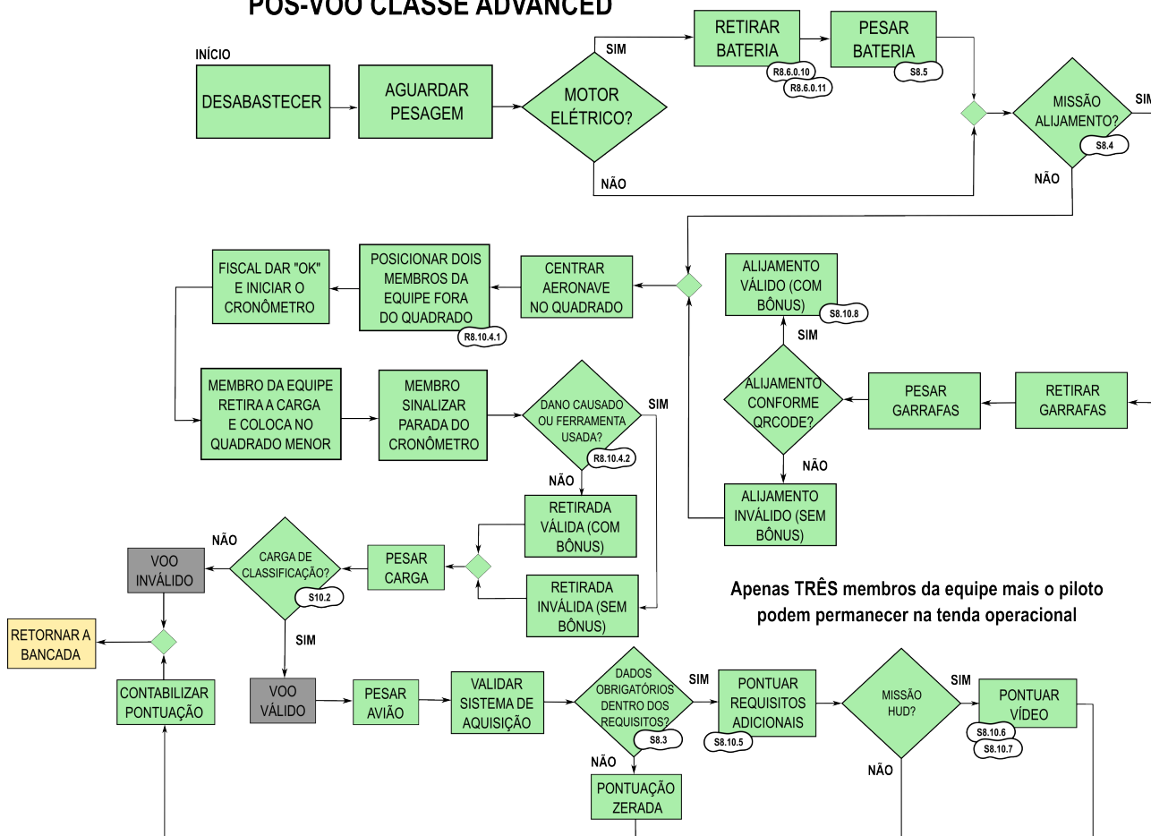
Figura 15.12: Pós-Voo - Classe Advanced
