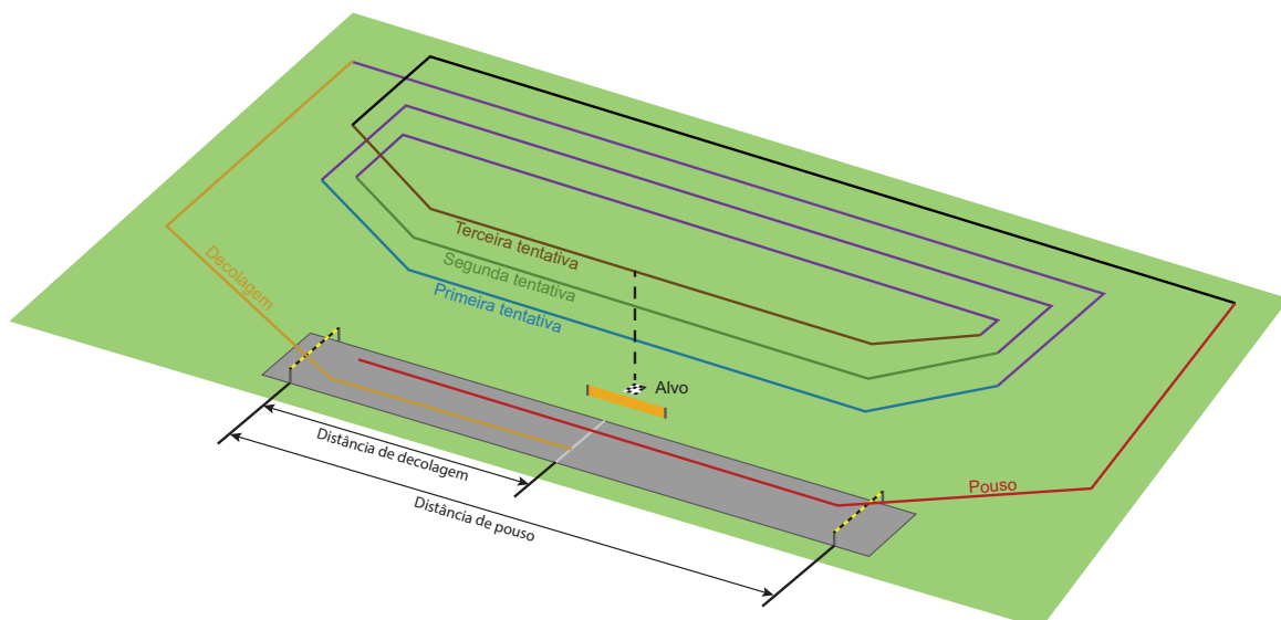
Figura 8.1: Exemplo de configuração possível.
